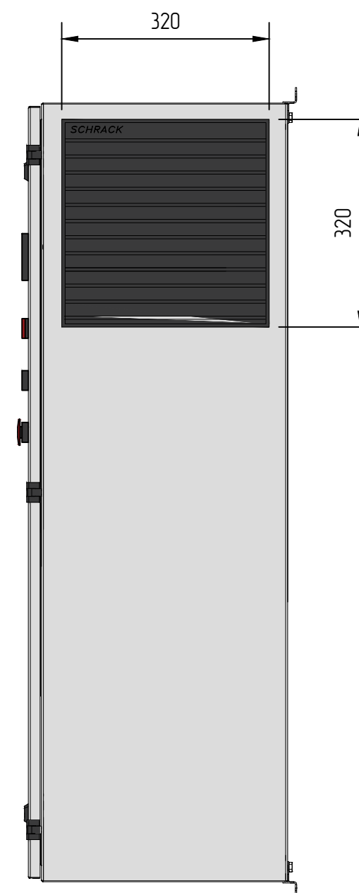
Вид справа
